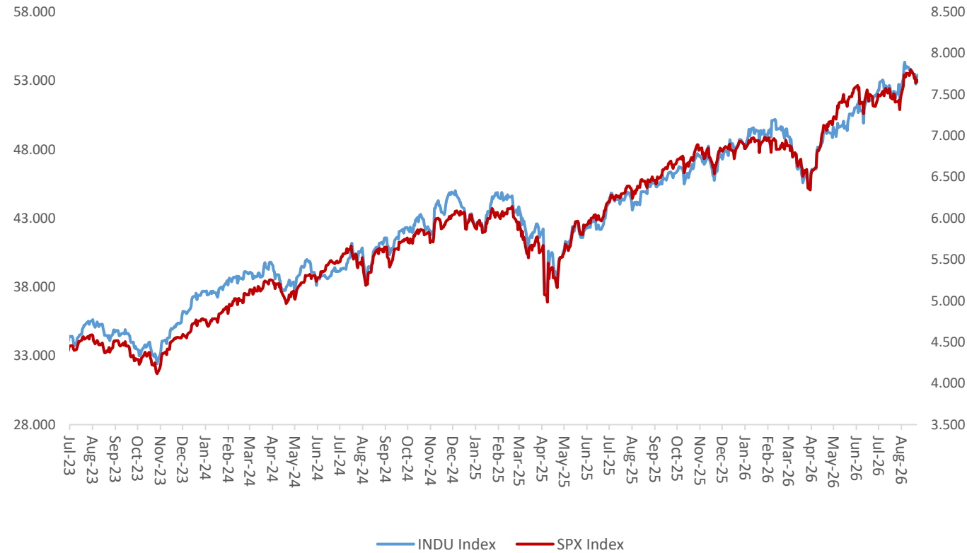
Grafik 4. DJIA & S&P 500 Index
